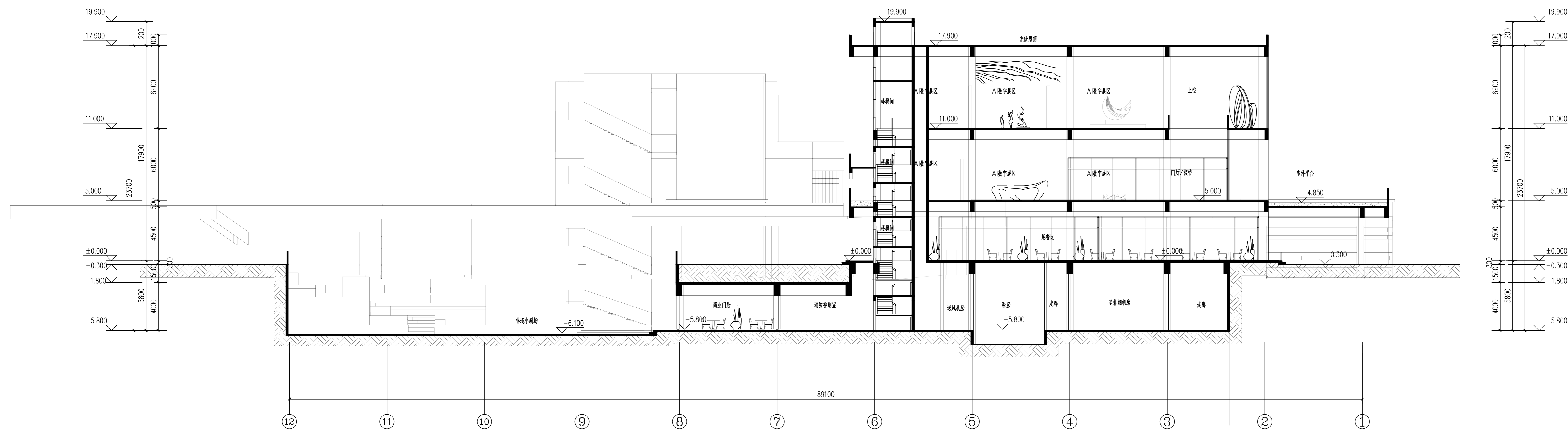
2-2剖面图 1:150
