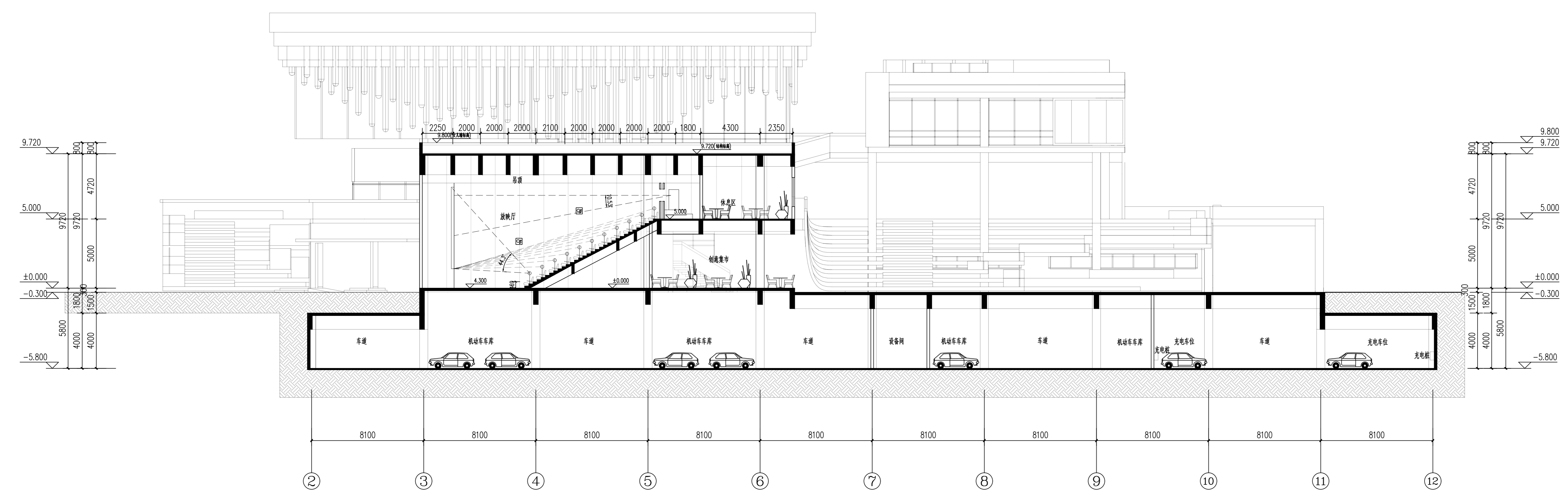
3-3剖面图 1:150
