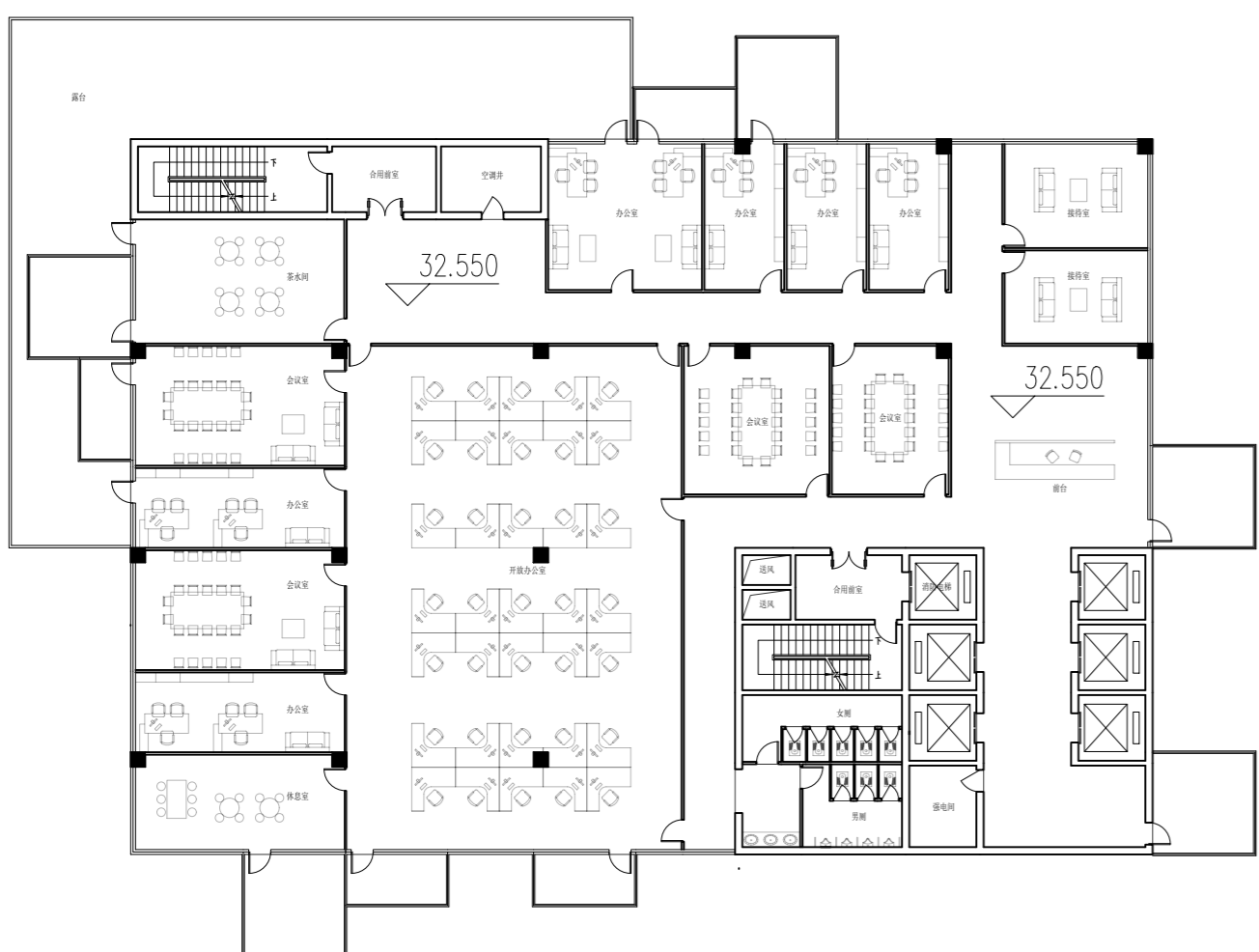
办公八层平面图 1:300
