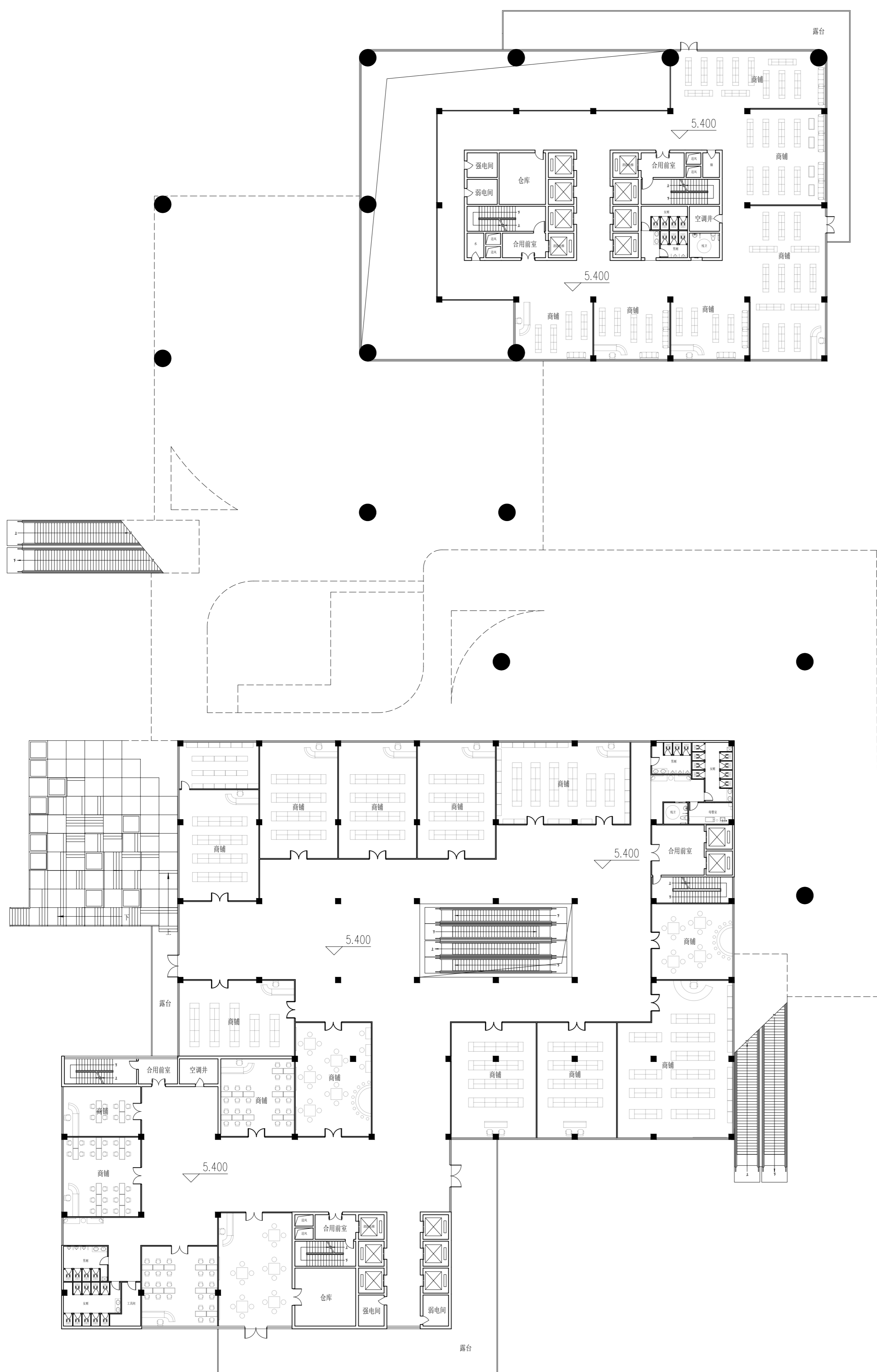
二层平面图 1:300
