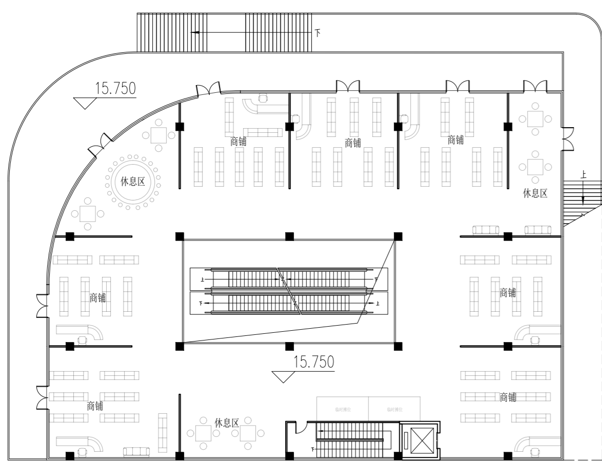
四层平面图 1:300
