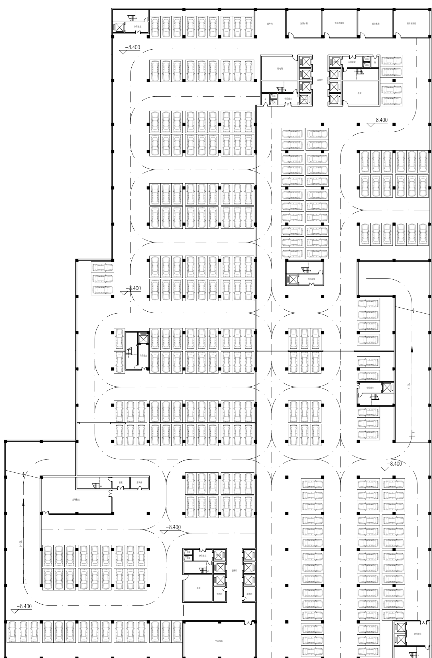
地下二层平面图 1:500
