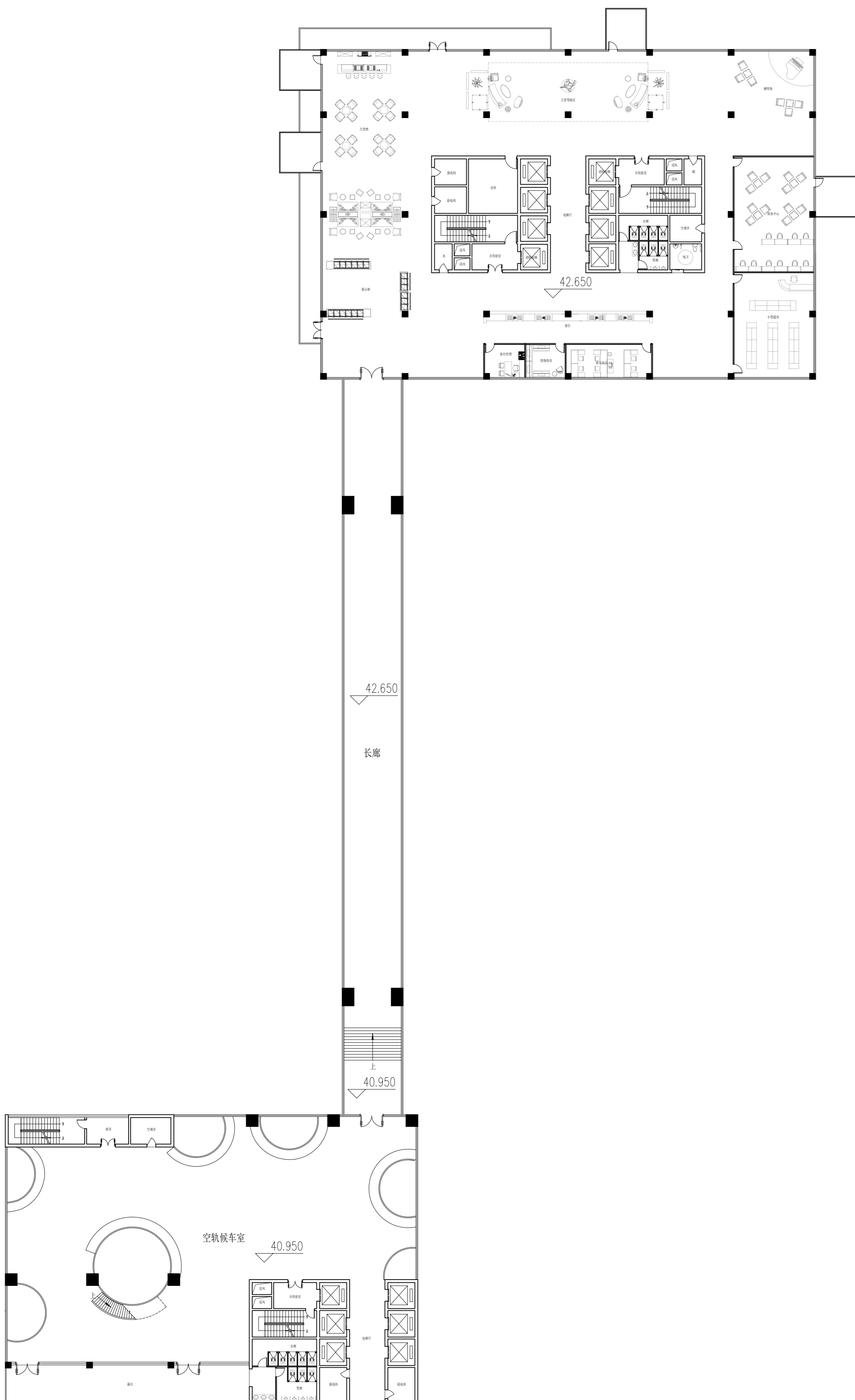
空轨大堂平面图 1:300
