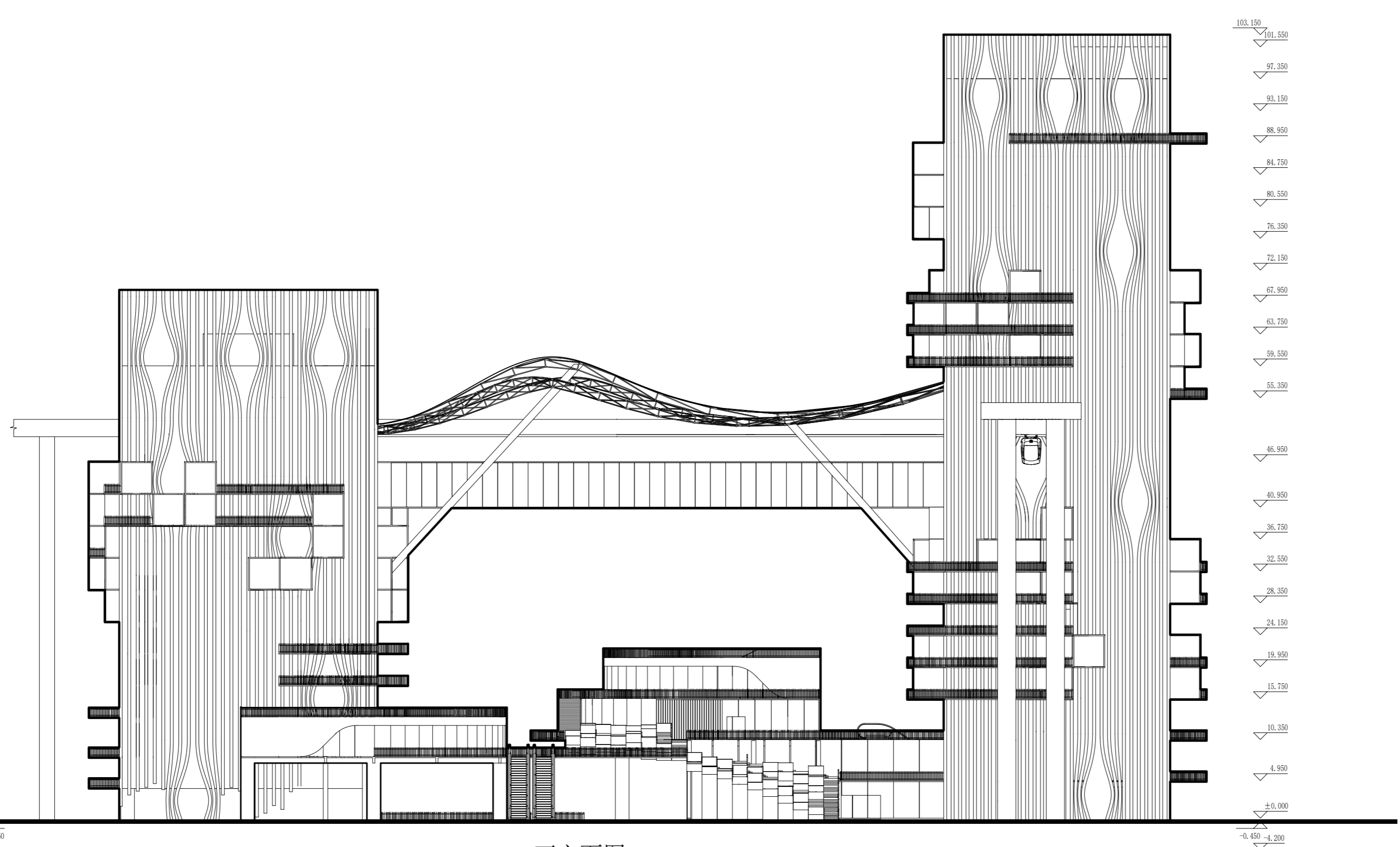
西立面图 1:500
