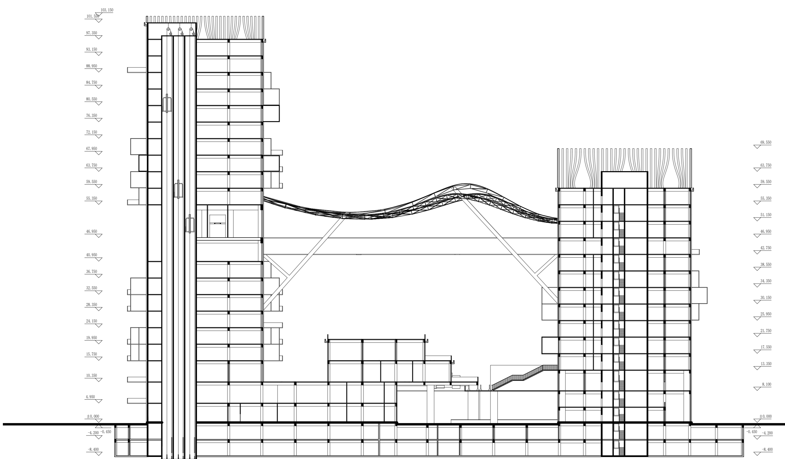
1-1剖面图 1:500
