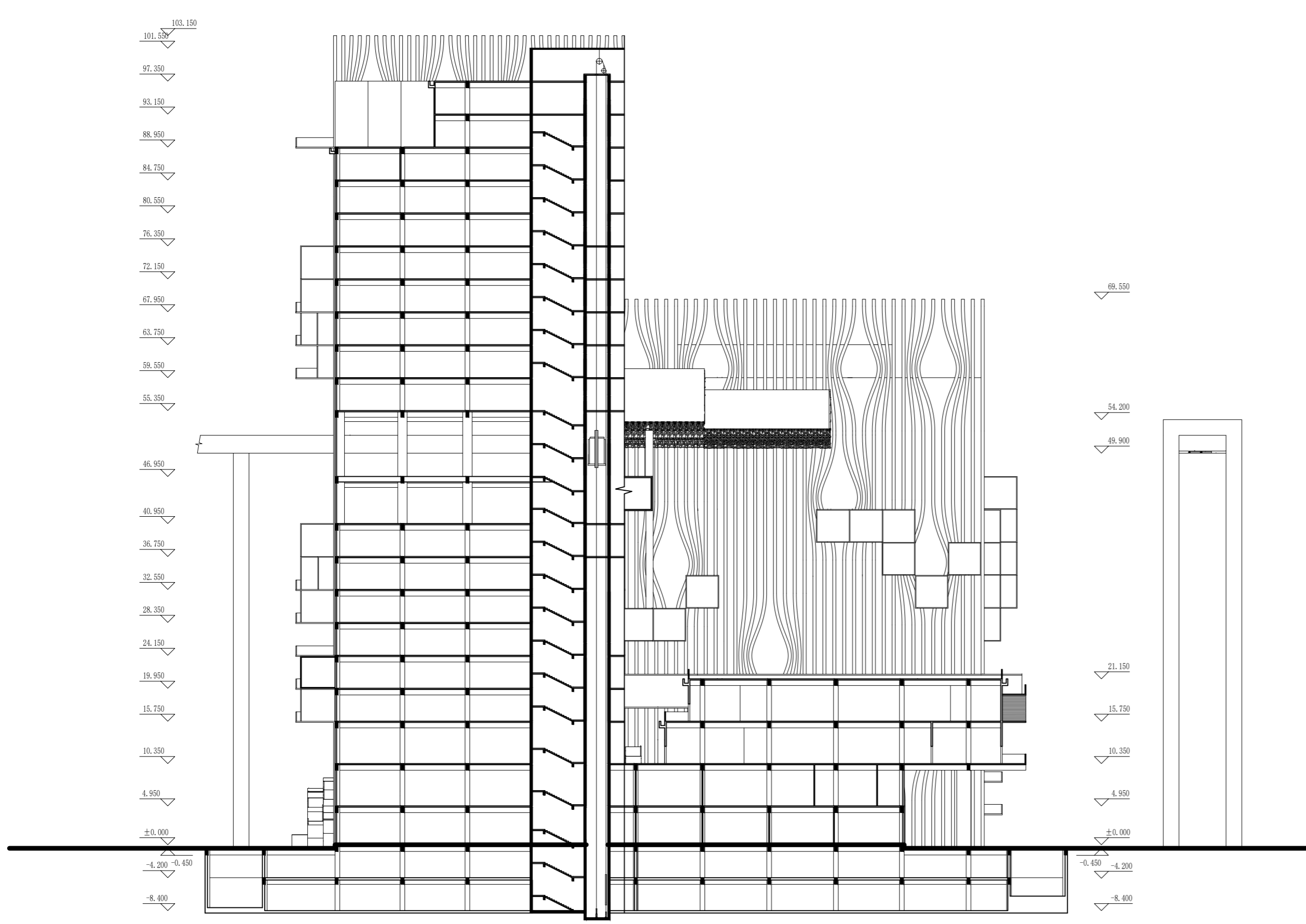
2-2剖面图 1:500
