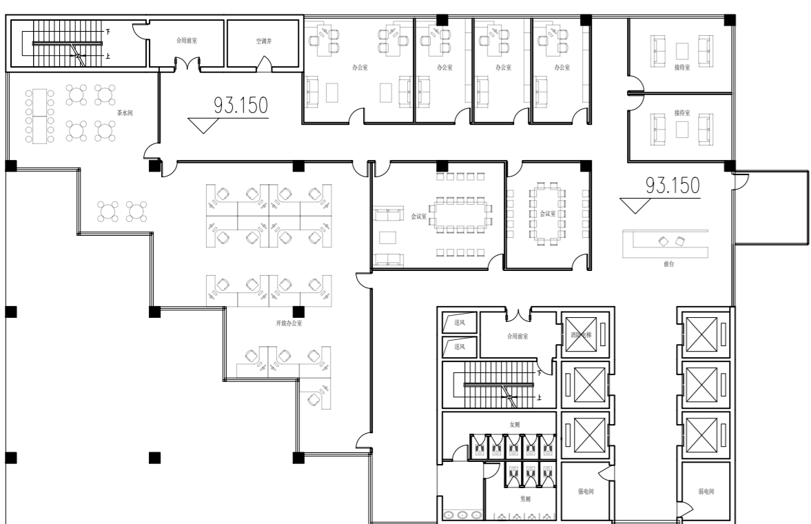
办公顶层平面图 1:300
